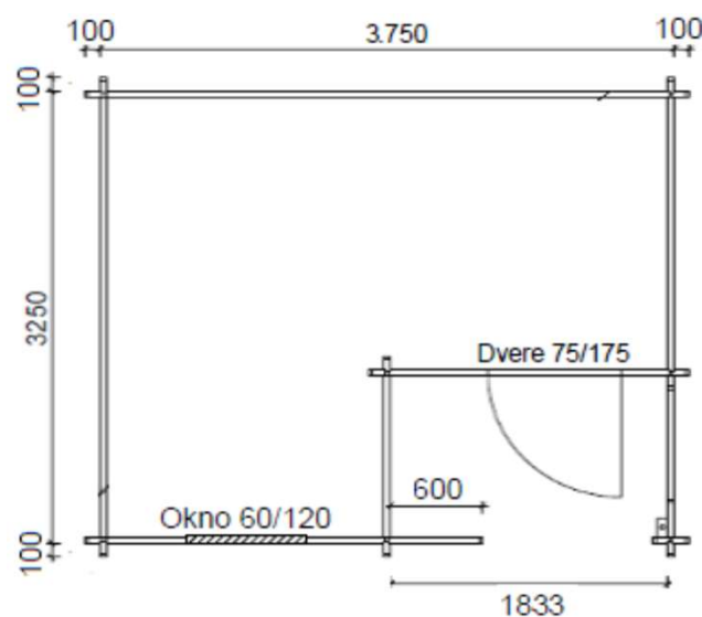
Pôdorys chatky:
